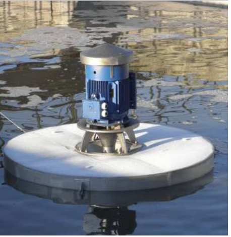
Dübalı Aerator Float Aerator
